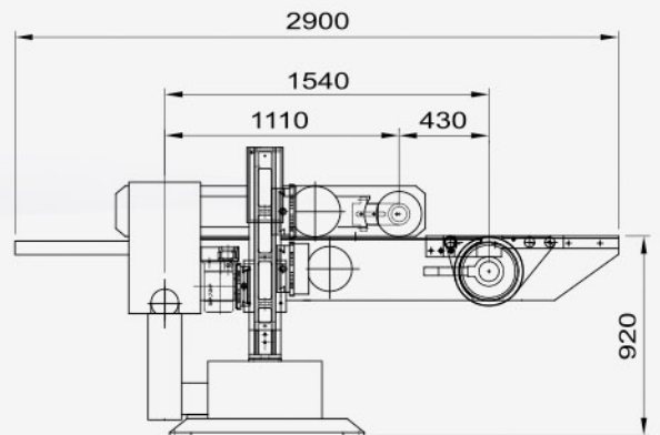
DET-E6-Model尺寸图
