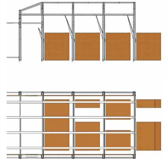
ÇOKLU BESLEME (Opsiyonel) MULTI FEED (Optional)
