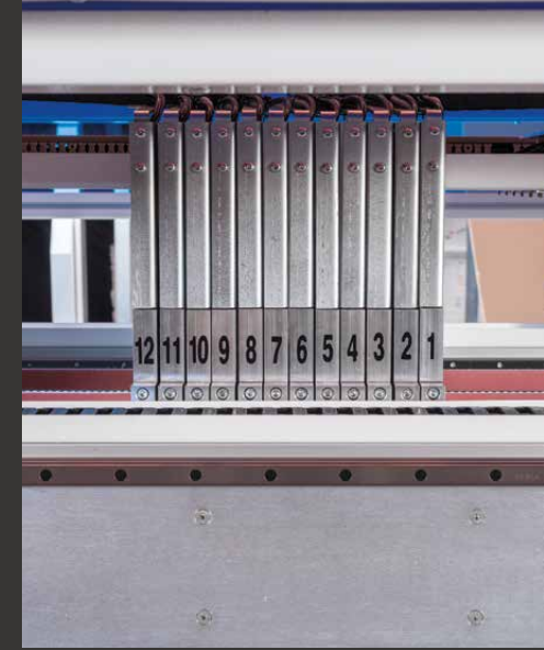
Opsiyonel 16 bıçağa kadar arttırılabilir. Optimal up to 16 blades.
